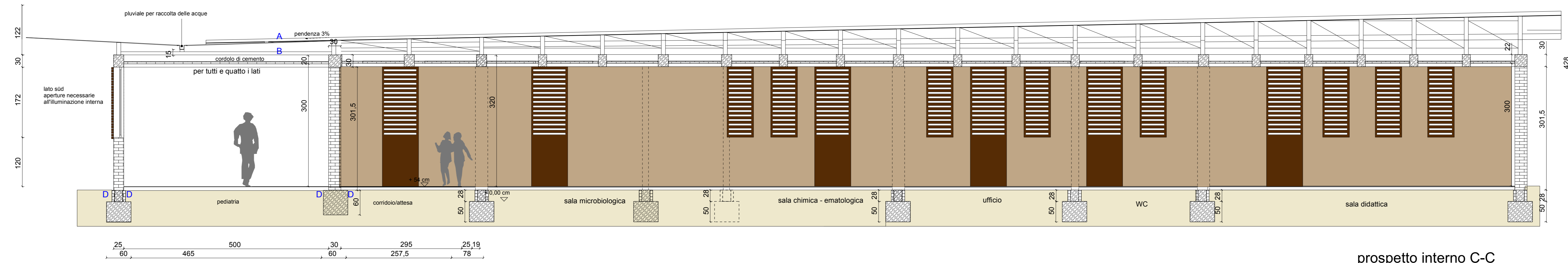
prospetto interno C-C
